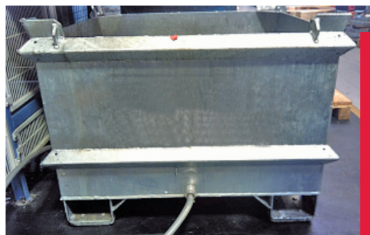
4 AUFFANGCONTAINER MIT DOPPELWANDIGEM BODEN, SPÄNESIEB UND ABLAßVORRICHTUNG FÜR EMULSIONEN
